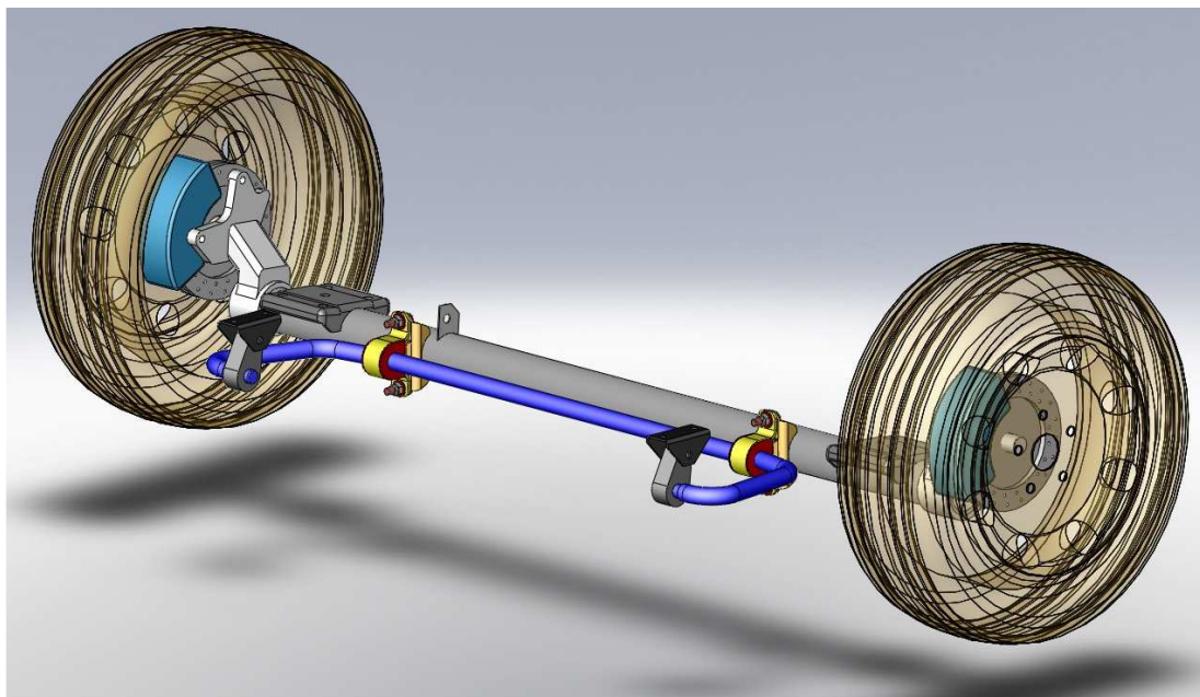
Représentation CAO d'un KIT BLEU arrière.
